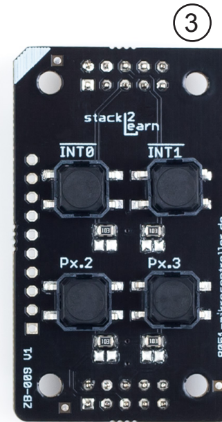
Bild 6. ZB-009 top
