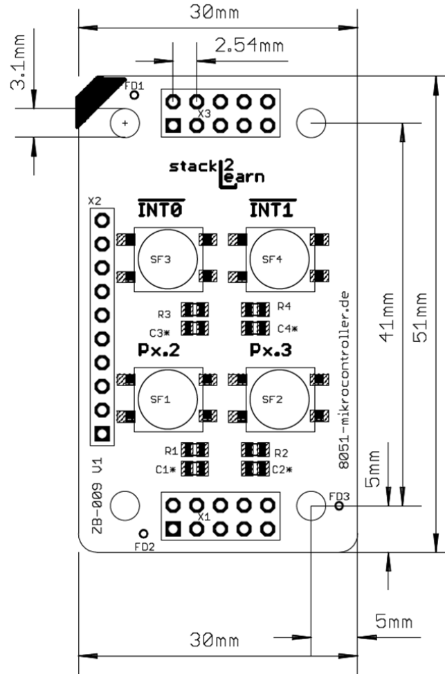
Bild 8. ZB-009 CAD Skizze bot
