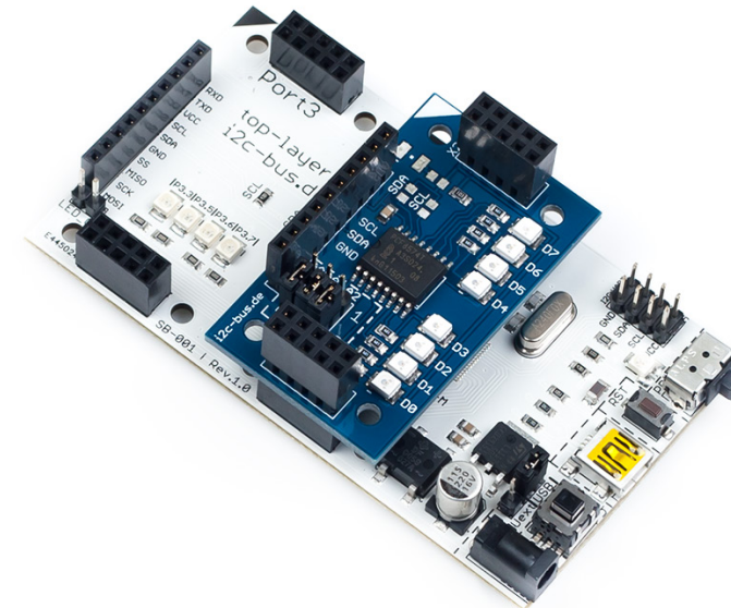
Bild 5. I2C-001 mit SB-001
