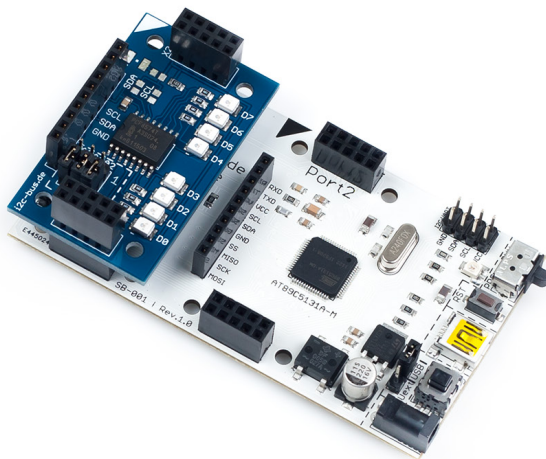
Bild 3. I2C-001 mit SB-001
