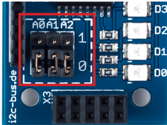
Bild 12. Slave Adresse Jumper
