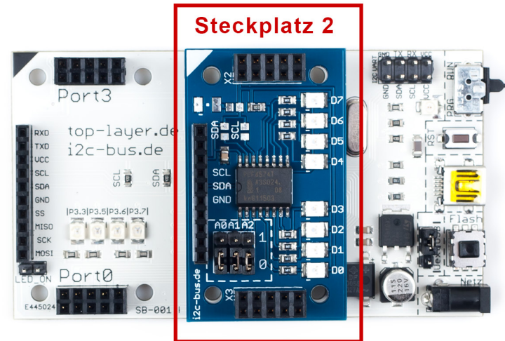
Bild 10. I2C-001 - Modul an Steckplatz 2
