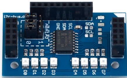
Bild 1. I2C-001 frontal Ansicht
