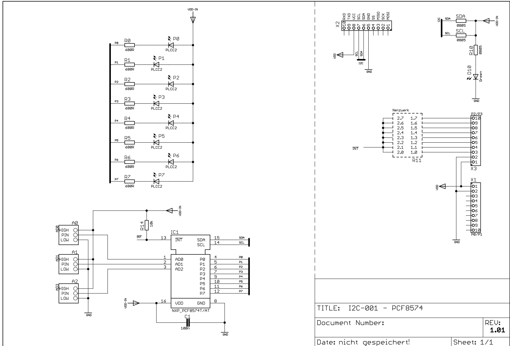
Bild 11. Schaltplan I2C-001
