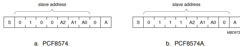
Bild 13. Slave Adresse (NXP Datenblatt Seite 9)
