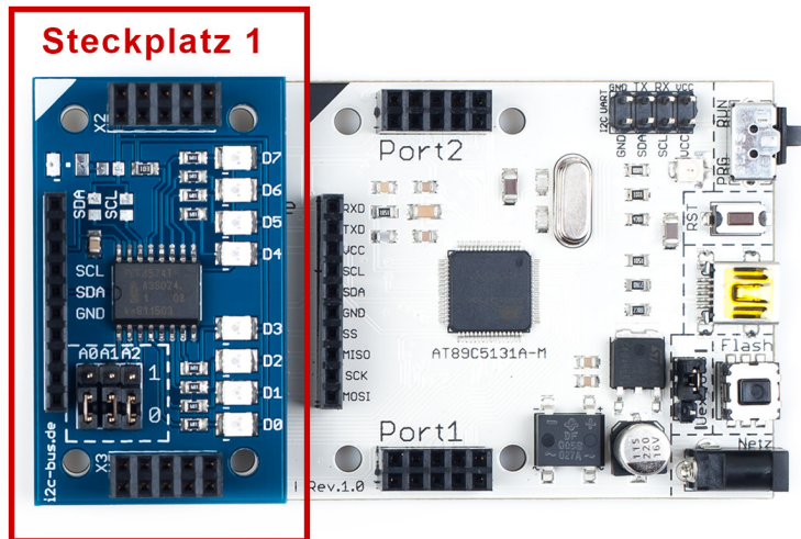
Bild 9. I2C-001 - Modul an Steckplatz 1
