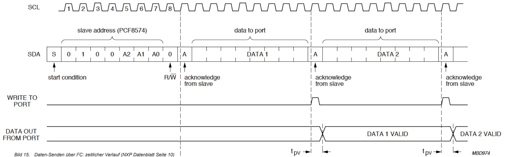
Bild 15. Daten-Senden über I 2 C: zeitlicher Verlauf (NXP Datenblatt Seite 10)
