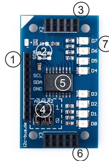
Bild 6. I2C-001 top
