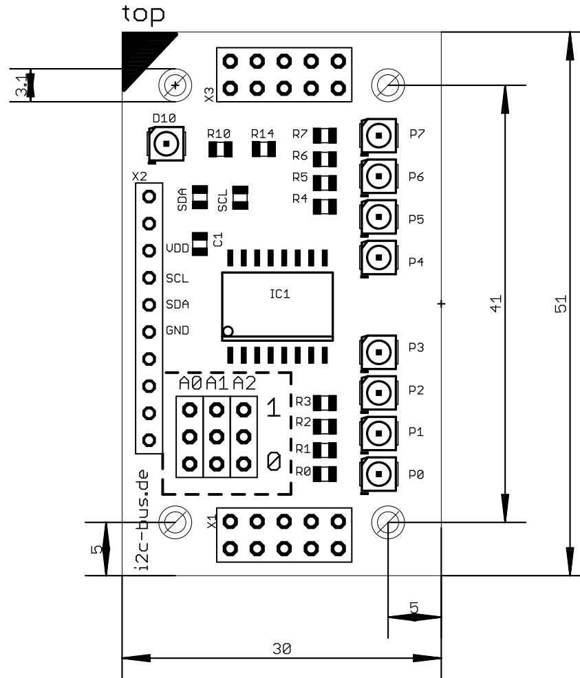
Bild 8. I2C-001 CAD Skizze top
